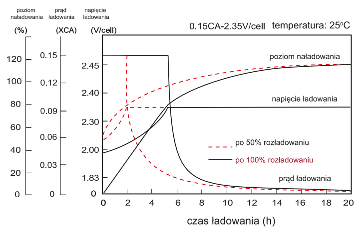
CHARAKTERYSTYKA ŁADOWANIA
