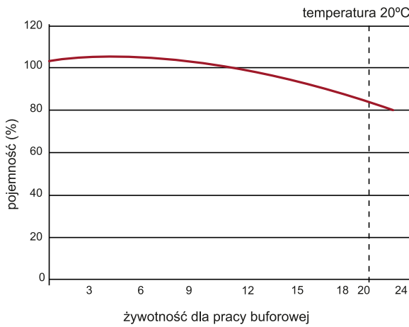
CHARAKTERYSTYKA POJEMNOŚCI AKUMULATORA
