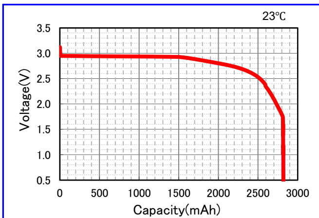
Discharge Curve (1kohm)
